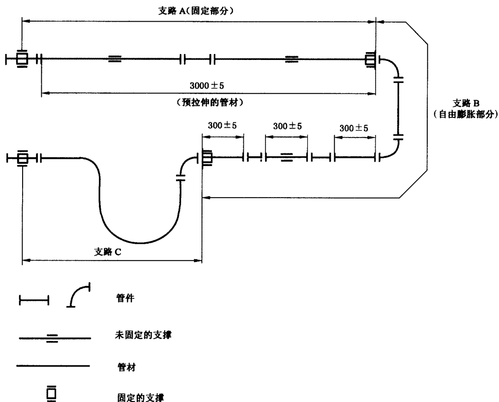
图 C.1 柔性管热循环试验组件安装示意图
