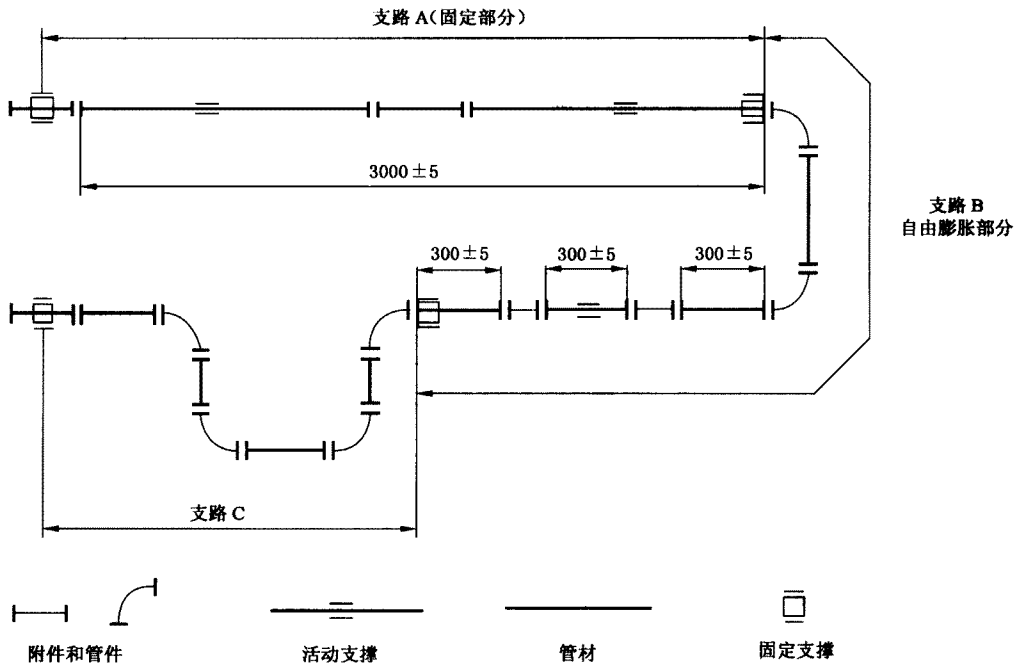
图 C.3 刚性管冷热水循环试验安装示意图
